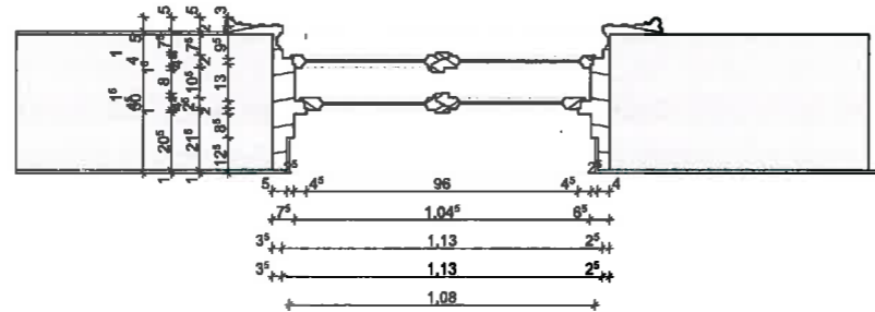
ALAPRAJZI NÉZET
